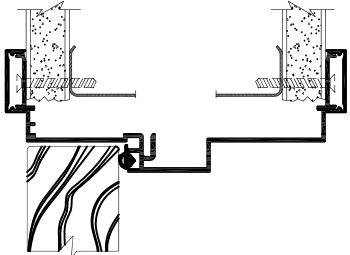
DOOR FRAME HEADER
